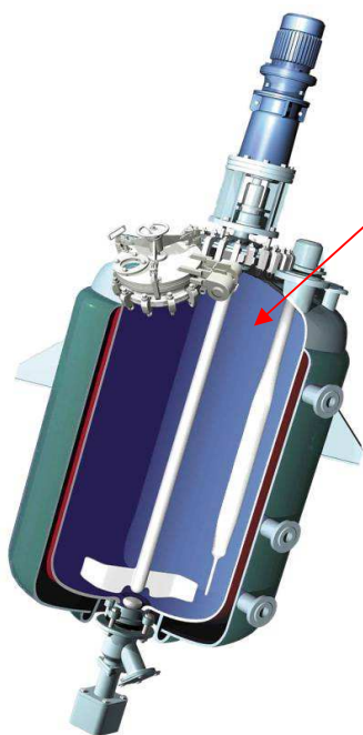
グラスライニング製反応機
