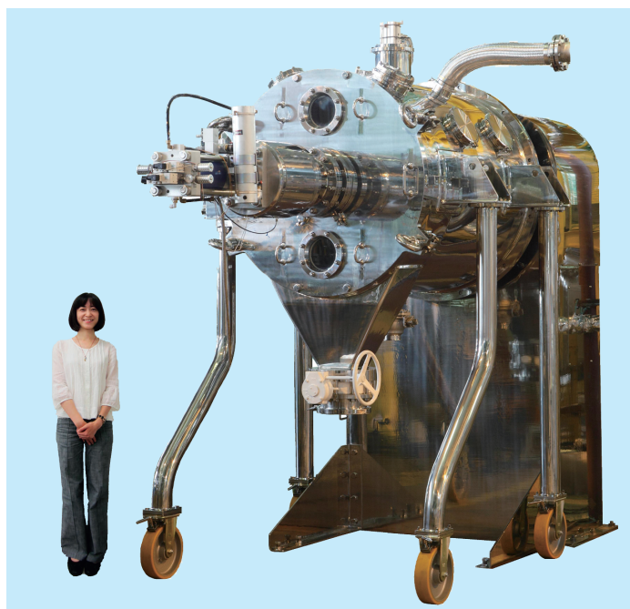
回転型ろ過乾燥機「RFD-1000」
