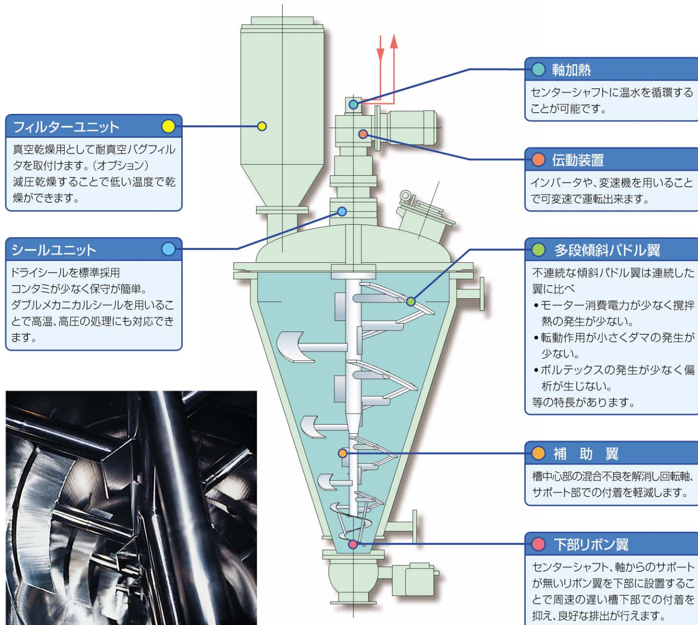
攪拌翼
