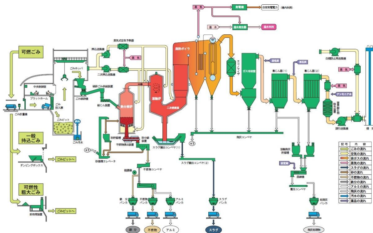
安芸クリーンセンター フロー図（現状）
